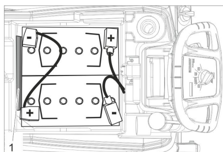
Bateria 6.654-093.0
